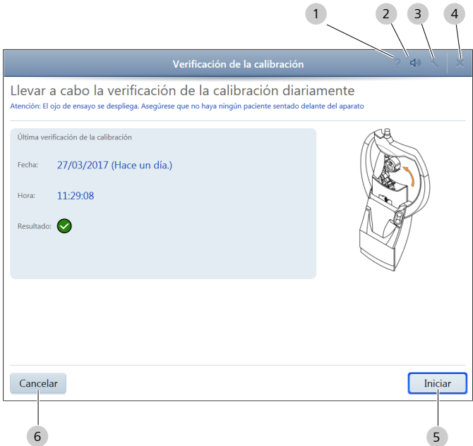
Fig. 8: Verificación de la calibración - Ventana de inicio
