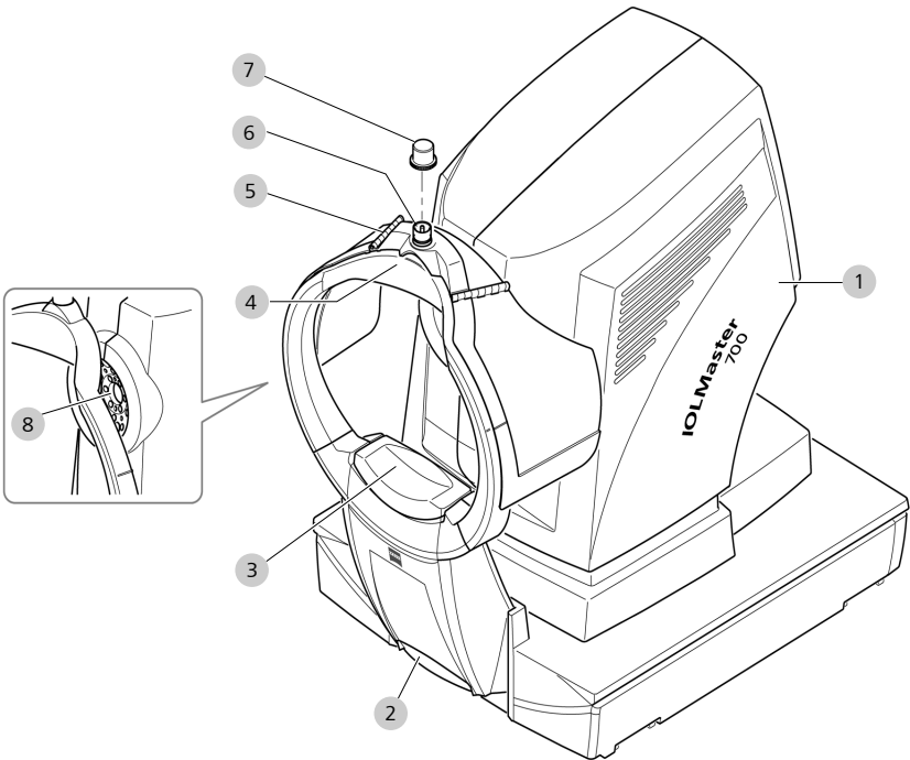
Fig. 3: Estructura del aparato, vista del lado del paciente
