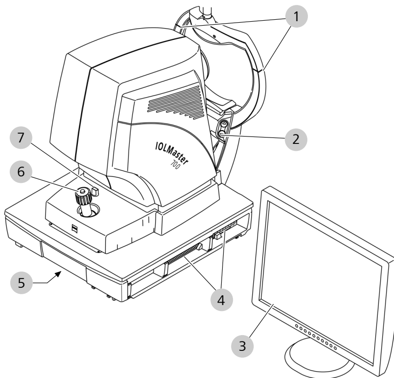
Fig. 2: Estructura del aparato, vista del lado del médico
