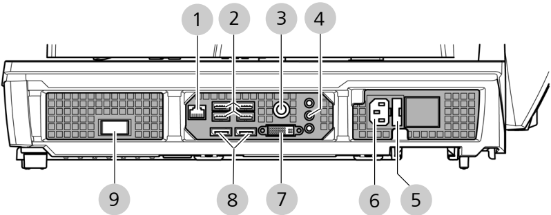
Fig. 4: Panel de conexiones del IOLMaster 700
