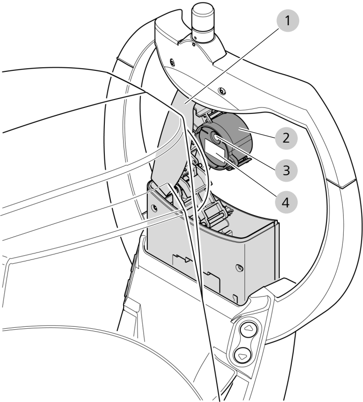
Fig. 10: Despliegue del soporte de la herramientas de ensayo
