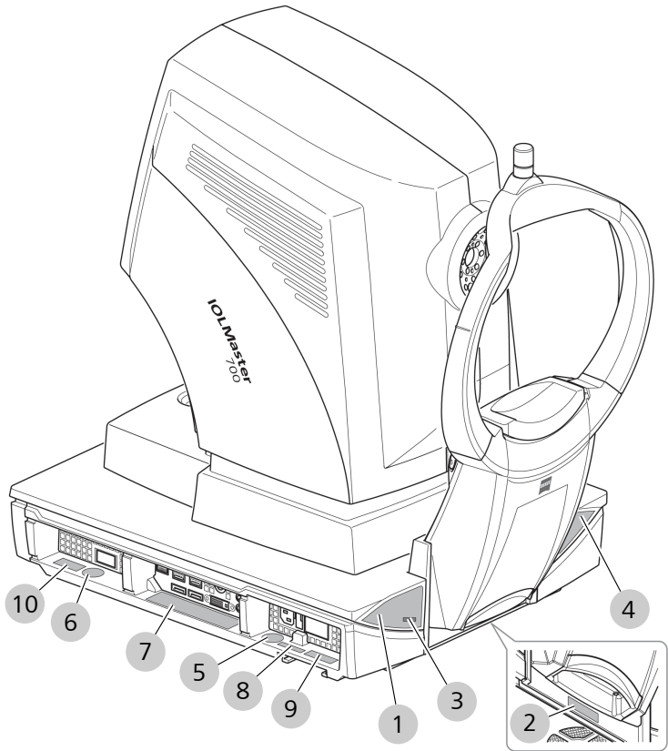
Fig. 1: Rótulos en el IOLMaster 700
