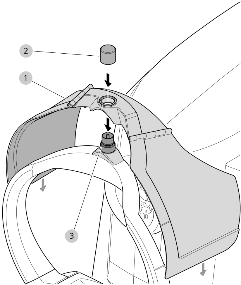
Fig. 7: Montaje de la cubierta contra luz dispersa para la opción Reference Image
