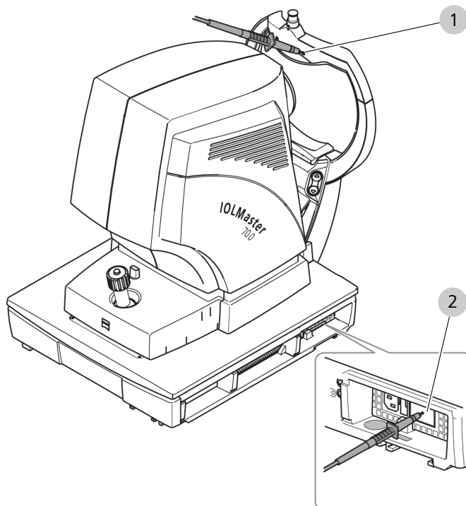
Fig. 83: Verificación de la seguridad eléctrica
