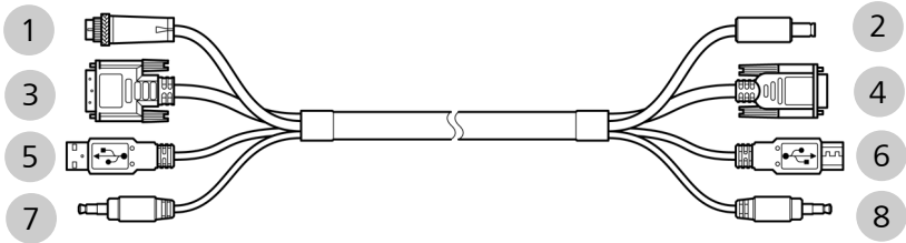
Fig. 6: Cable de conexión Operator Interface
